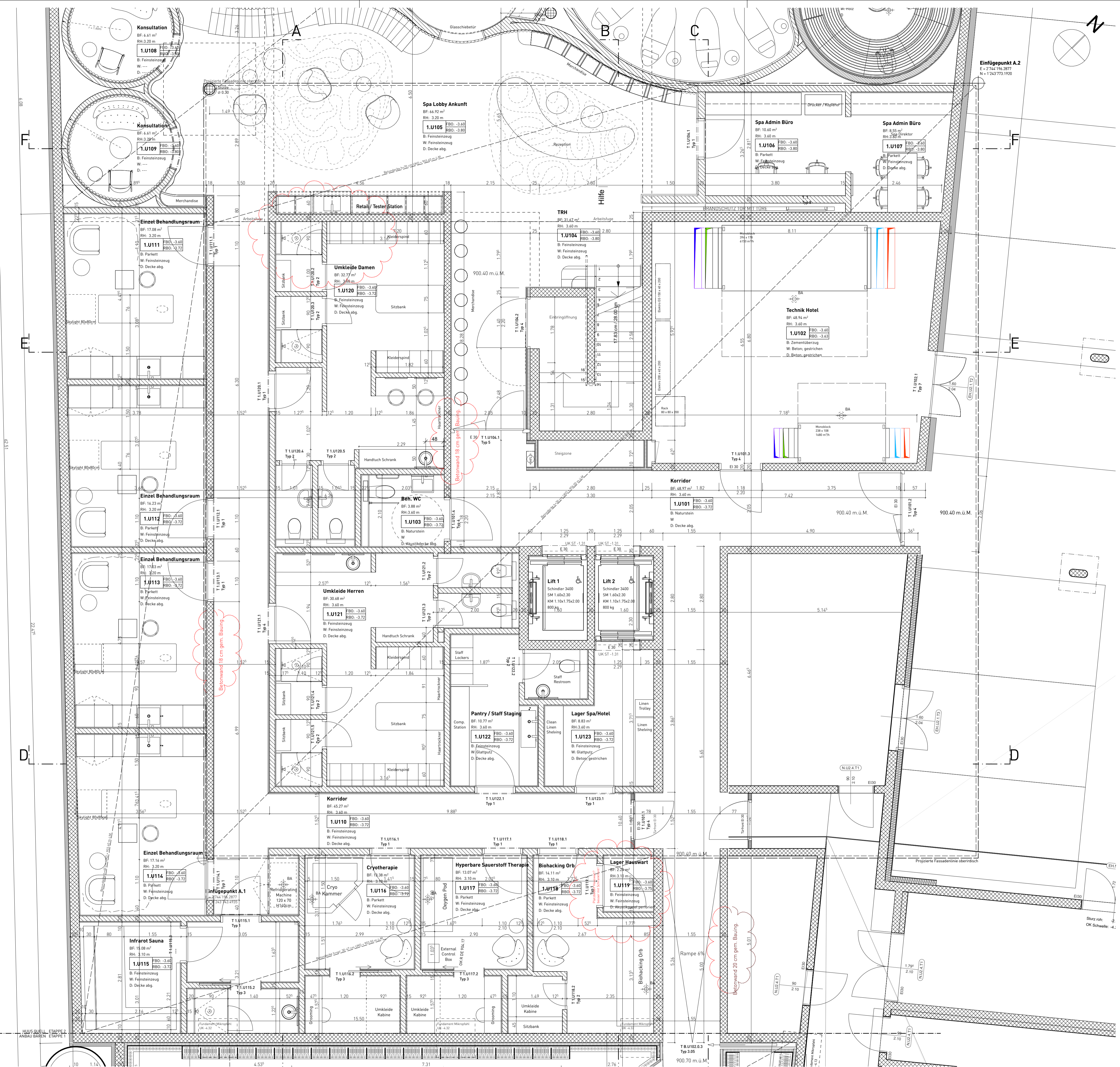
HAUS 1 1. UG 1:50
